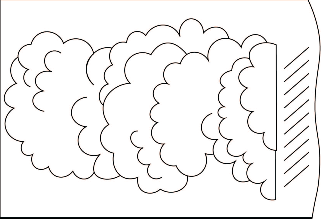
cumulonimbus
