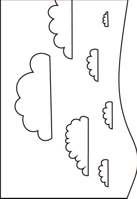
cumulus
