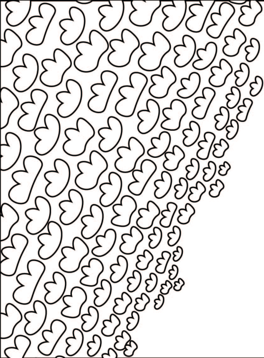
altocumulus
