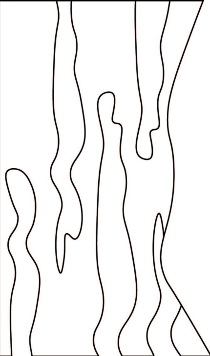
altocumulus
